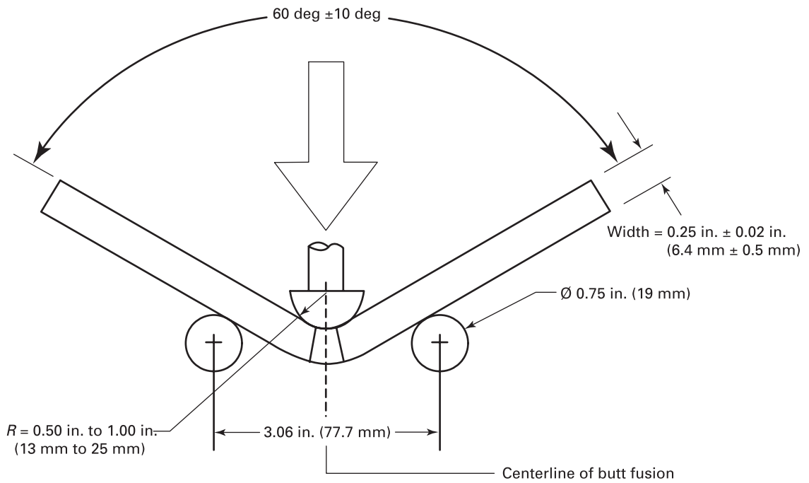
(d) Guided Side-Bend Test Machine Dimensions
